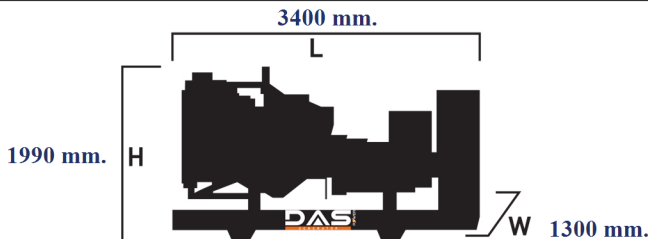
Islak Ağırlık: 3300 kg. Yakıt Tankı Kapasitesi: 295 L
