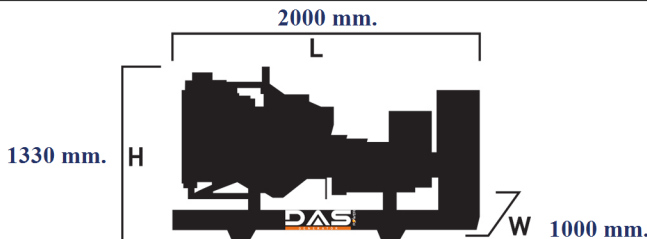
Islak Ağırlık: 1100 kg. Yakıt Tankı Kapasitesi: 138 L
