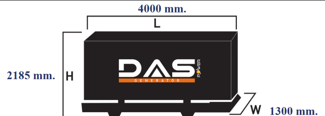
Islak Ağırlık: 3850 kg. Yakıt Tankı Kapasitesi: 295 L
