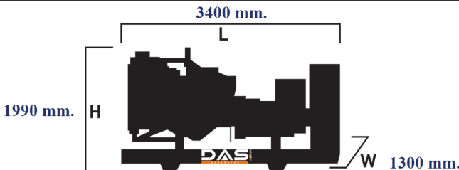
Islak Ağırlık: 2965 kg. Yakıt Tankı Kapasitesi: 295 L
