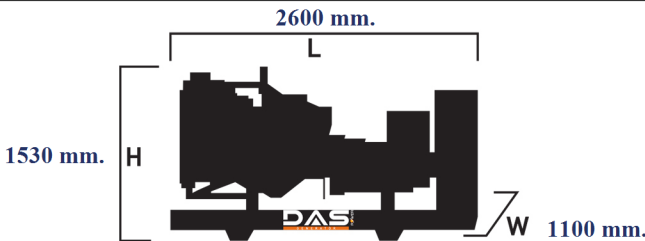
Islak Ağırlık: 1700 kg. Yakıt Tankı Kapasitesi: 173 L
