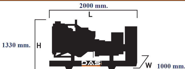
Islak Ağırlık: 1000 kg. Yakıt Tankı Kapasitesi: 138 L
