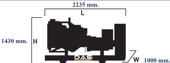
Islak Ağırlık: 870 kg. Yakıt Tankı Kapasitesi: 138 L
