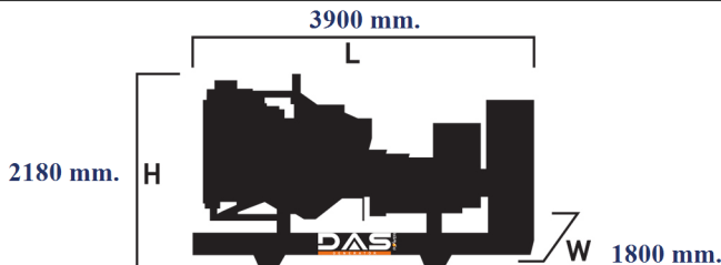
Islak Ağırlık: 4080 kg. Yakıt Tankı Kapasitesi: 495 L
