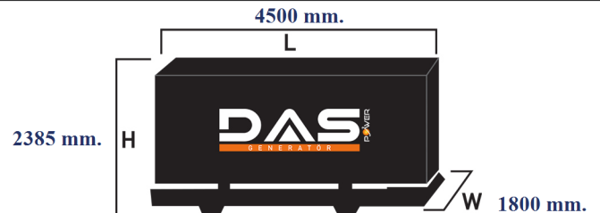
Islak Ağırlık: 5690 kg. Yakıt Tankı Kapasitesi: 495 L
